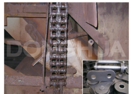
24. Steel mill balance chain Ausgleichsketten für die Stahlindustrie
