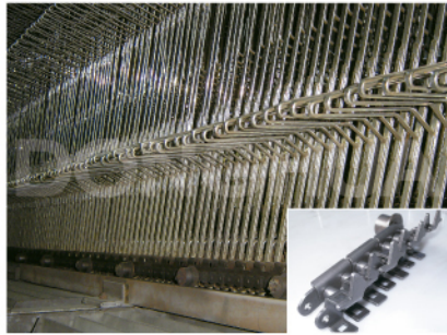
26. Conveyor chain for drying room Rollenketten für Lackier- und Trocknungsanlagen
